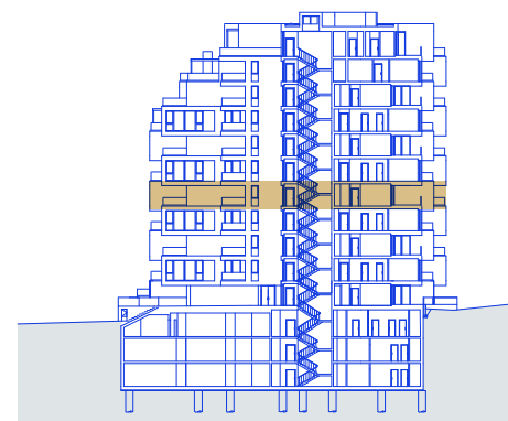
ŘEZ OBJEKTEM
