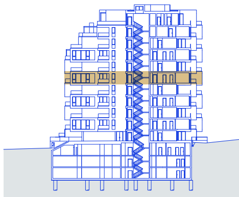
ŘEZ OBJEKTEM
