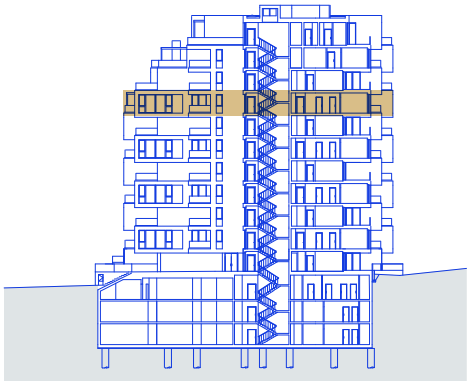
ŘEZ OBJEKTEM
