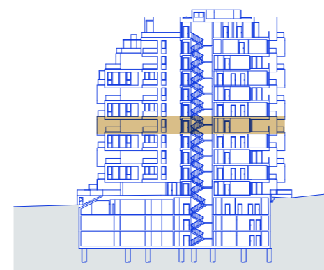
ŘEZ OBJEKTEM
