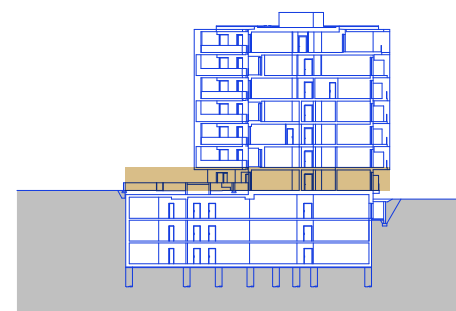
ŘEZ OBJEKTEM
