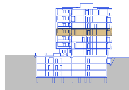
ŘEZ OBJEKTEM
