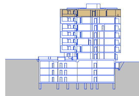
ŘEZ OBJEKTEM
