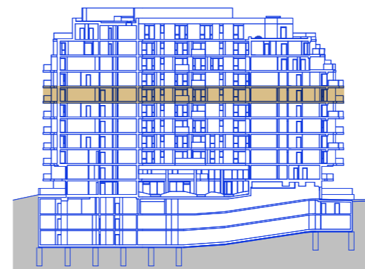
řez objektem
