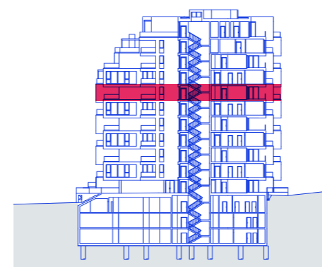
ŘEZ OBJEKTEM
