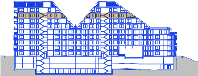
řez objektem
